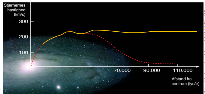
Figur 2 – Stjernernes observerede banehastigheder (fuldttrukken linie) i vores nærmeste nabogalakse, Andromeda, følger ikke den teoretiske forudsigtelse (stiplede linie). At stjerner ikke slynges ud i rummet kan forklares med et bidrag til tyngdekraften fra mørkt stof.
