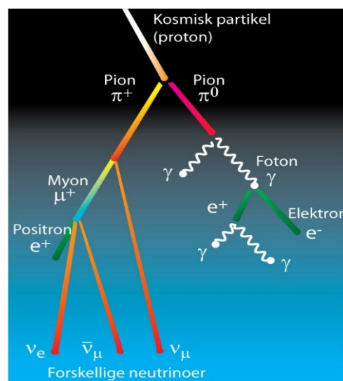
Illustration af partikelbyge (fra artiklen).
